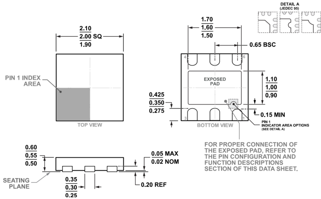
图 29.6 引脚 DFN-6
