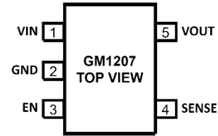
图 4.3 引脚 SOT-23 引脚配置
