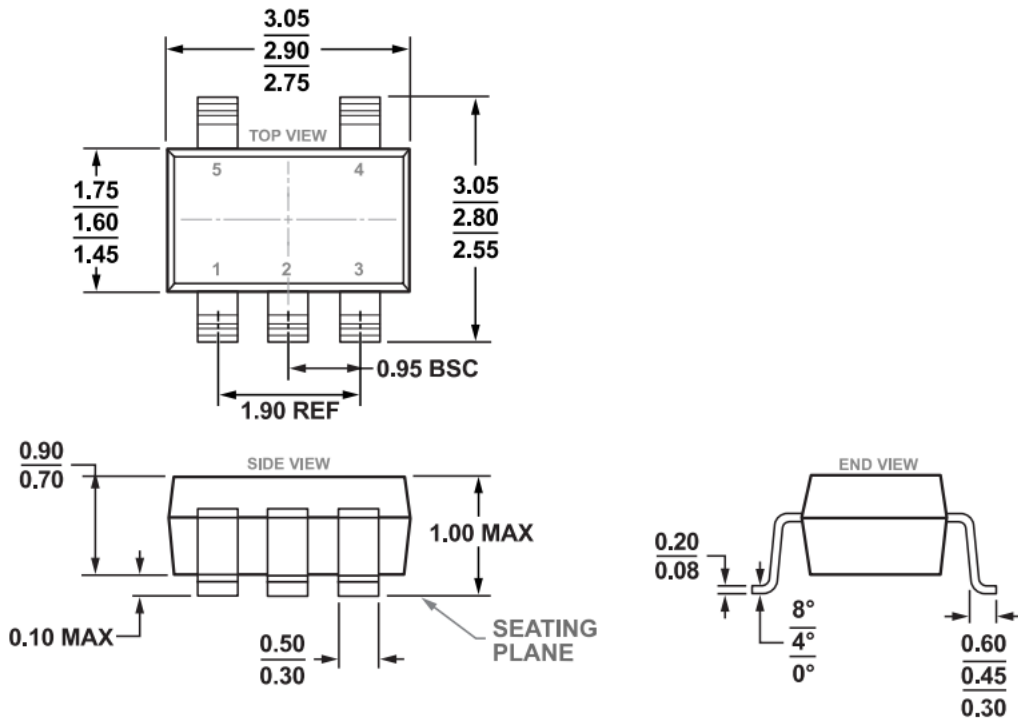
图 30.5 引脚 SOT-23
