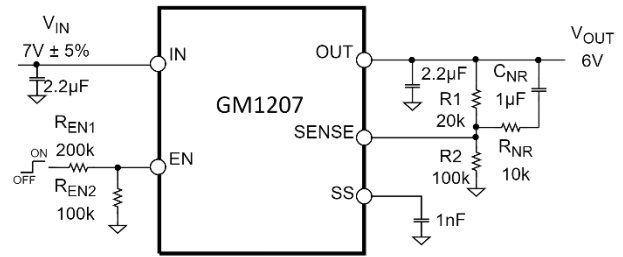
图 28. 噪声优化
