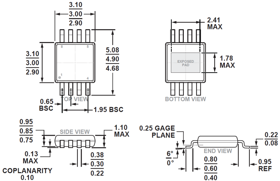
图 32.8 引脚 MSOP
