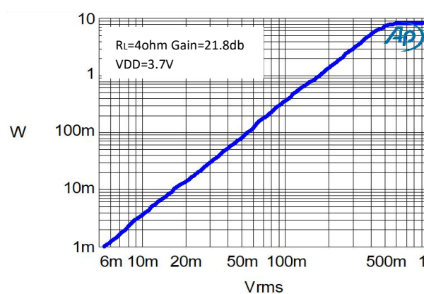
Vin vs Output Power
