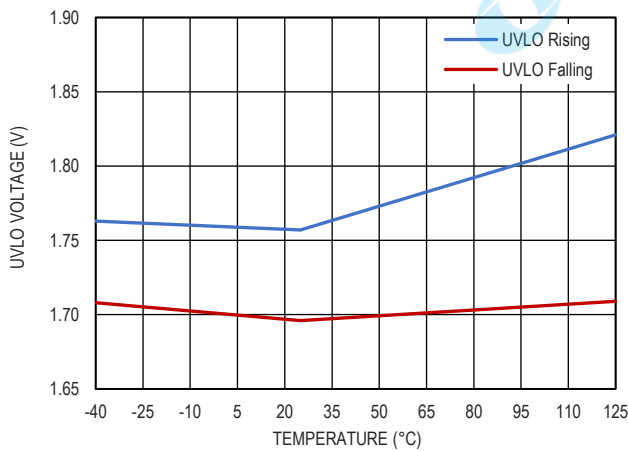
图 14. UVLO 阈值
