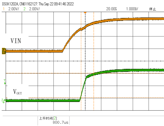
图 18. 软启动, V_{IN}=5.5V , V_{OUT}=5.0V , I_{OUT}=1.5A
