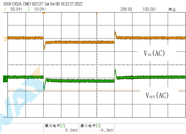
图 19. 负载瞬态响应, V_{IN}=2.8V , V_{OUT}=1.8V , I_{OUT}=100mA to 1.5A
