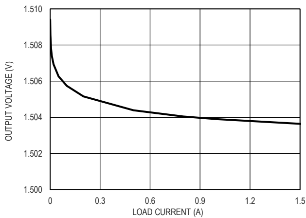
图 8. 1.5V 输出电压和负载电流的关系
