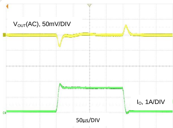
图 15. V_{OUT} = 1.2V , I_O = 0.1A 至 1.6A , FPWM 模式
