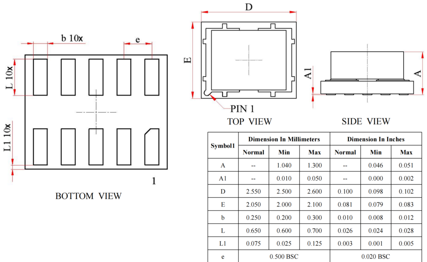
图 18.8 引脚 LGA (2.0mm x 2.5mm)
