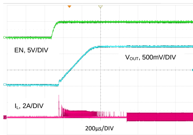
图 12. 启动波形, V_{OUT} = 1.2\text{V} , I_o = 10\text{mA}
