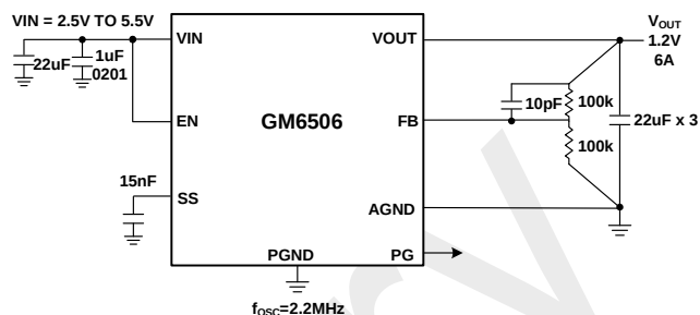
图 1. GM6506 典型应用
