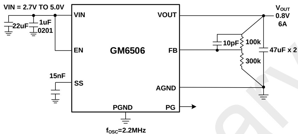
图 17. V_{IN}=3.3V , V_{OUT}=0.6V , I_{LOAD}=6A
