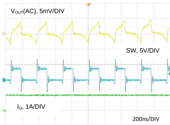
图 14. V_{OUT} = 1.2V , I_O = 1A , FPWM 模式
