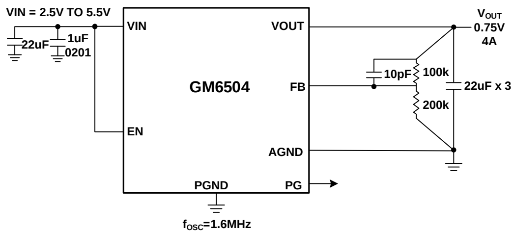
图 17. V_{IN}=3.3V , V_{OUT}=0.75V , I_{LOAD}=4A
