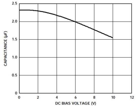
图 25. 电容与电压关系特性
