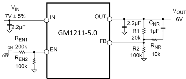
图 26. 噪声优化
