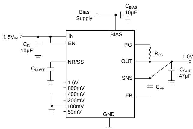
图 1 GM1503-1 典型应用
