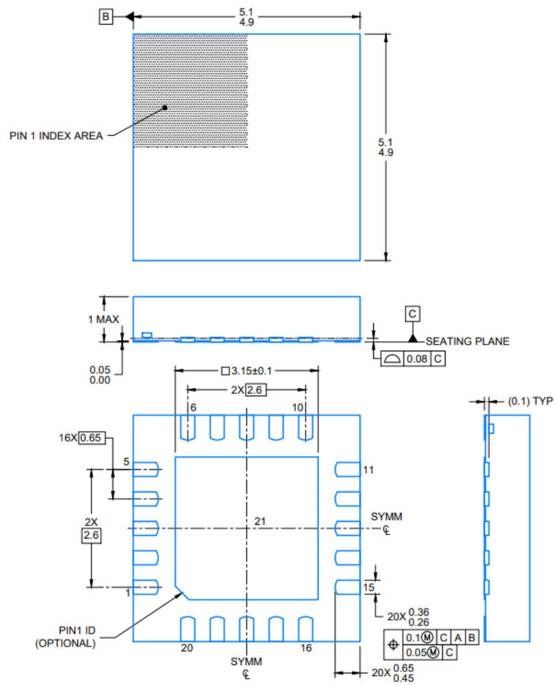
图 32. 20 引脚 QFN (5 毫米 x 5 毫米)
