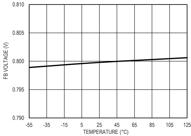
图 7. FB 引脚电压和温度的关系
