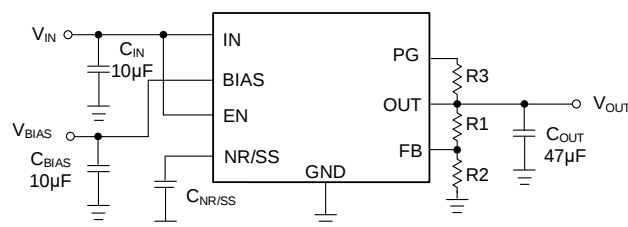
图 2 GM1503-2 典型应用
