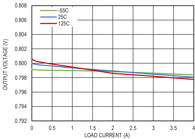
图 9. 负载调整率, V_{BIAS} = 5V
