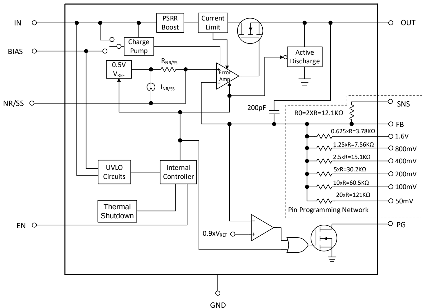
图 3. GM1503-1 方框图
