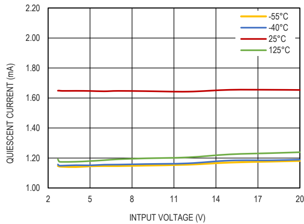
图 11. 静态电流和输入电压的关系, I_{OUT}=1mA
