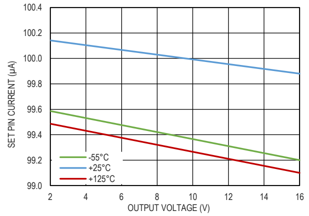
图 6. SET pin 电流和输出电压的关系
