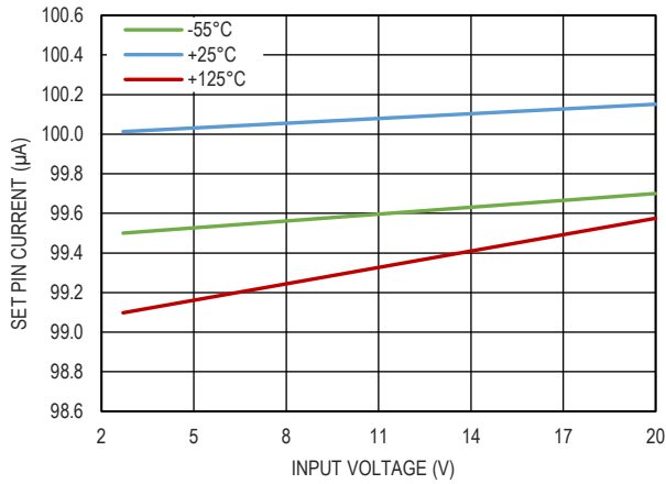
图 5. SET pin 电流和输入电压的关系
