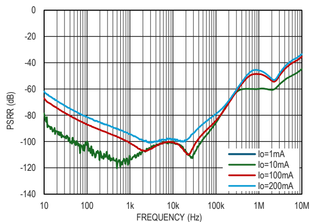
图 20. 电源电压纹波抑制比, V_{IN}=4.3V , V_{OUT}=3.3V
