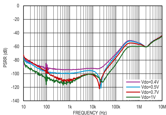
图 19. 电源电压纹波抑制比和压差的关系, I_{OUT}=10mA
