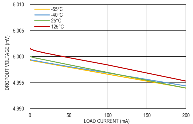
图 10. V_{OUT} = 5.0V 时的负载调整率
