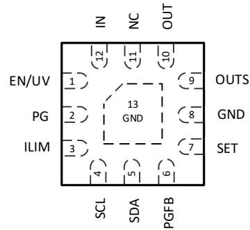
图 3. QFN 引脚配置(顶视图)
