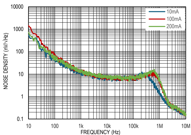
图 18. 输出噪声谱密度, V_{IN}=4.3V , V_{OUT}=3.3V
