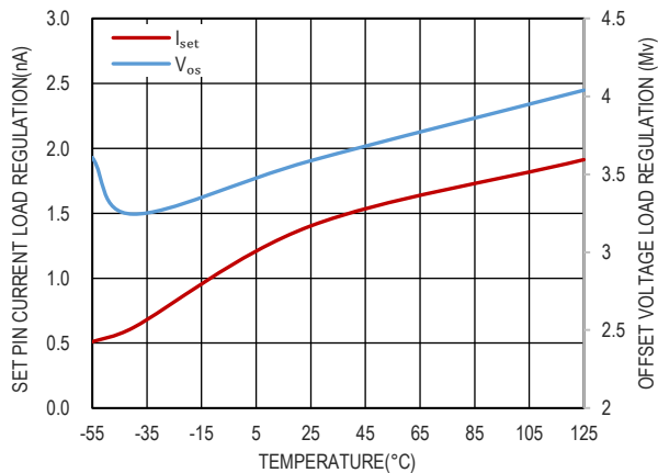
图 9. SET pin 电流、 |V_{OUT} - V_{SET}| 和温度的关系
