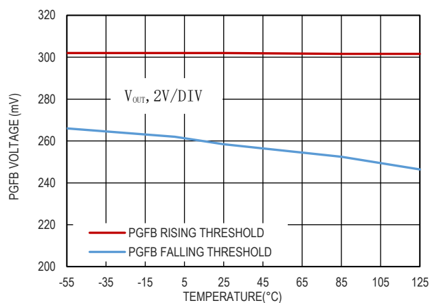
图 17. PGFB pin 阈值
