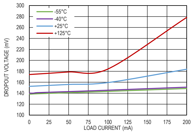
图 13. 压差电压和负载电流的关系, V_{OUT}=5.0V
