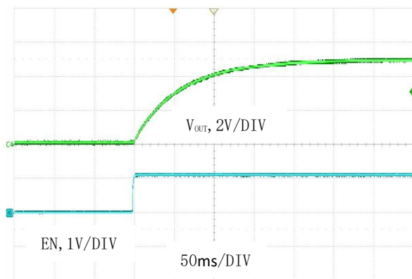
图 21. 软启动, V_{IN}=5.7V , V_{OUT}=5.0V , I_{OUT}=200mA
