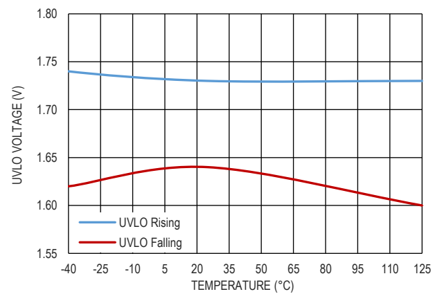
图 14. UVLO 阈值
