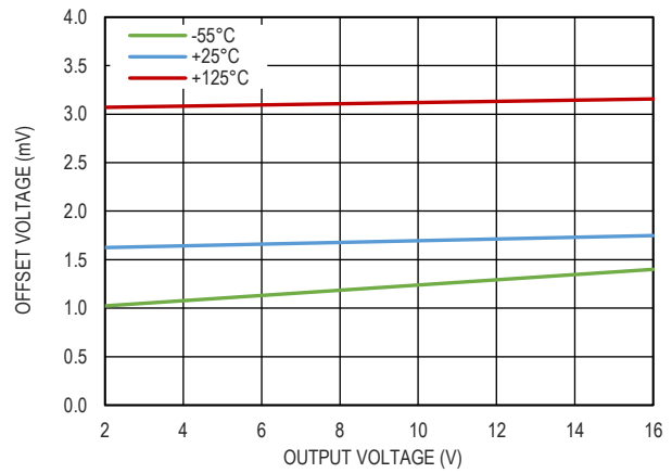
图 8. |V_{OUT} - V_{SET}| 和输出电压的关系
